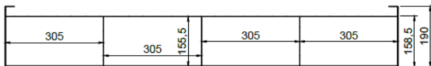
SEZIONE A-A
